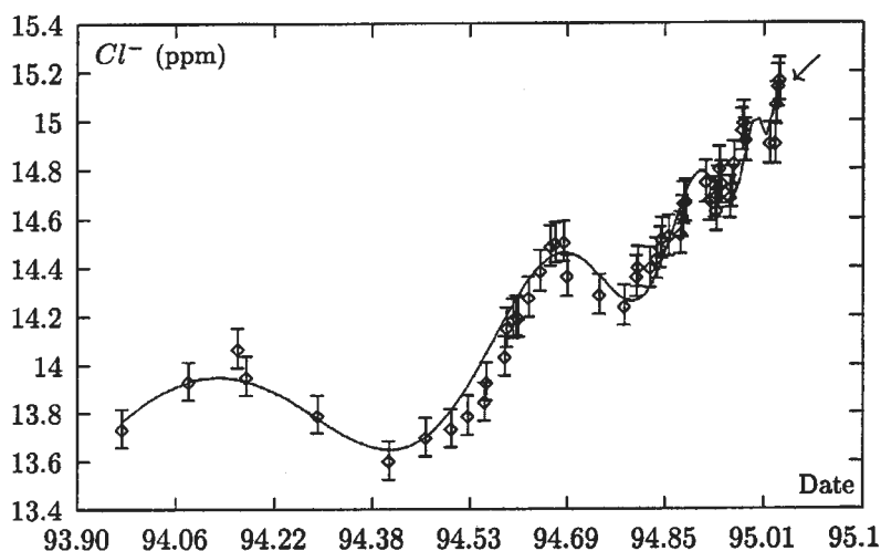
Рисунок 3. КОНЦЕНТРАЦИЯ ИОНОВ ХЛОРА В ПОДЗЕМНЫХ ИСТОЧНИКАХ ПЕРЕД ЗЕМЛЕТРЯСЕНИЕМ В КОБЕ (17.01.1995)
